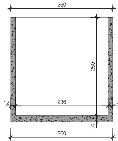
Dwarsdoorsnede
