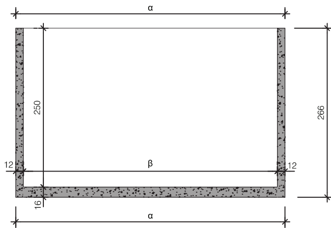
Langsdoorsnede
